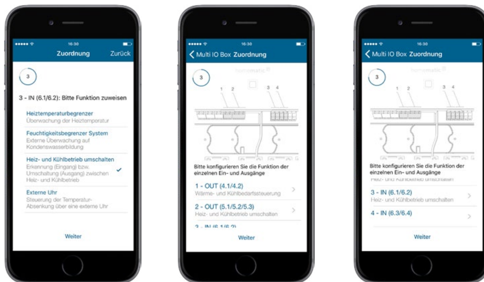
Abbildung 43: Screenshot Konfiguration Multi IO Box für Wechsel zwischen Heiz- und Kühlbetrieb über einen extern angeschlossenen Schalter (2)
