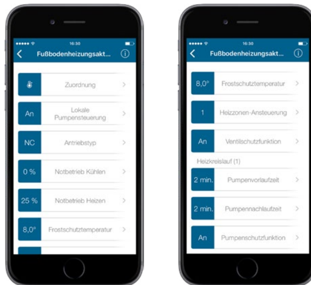
Abbildung 35: Screenshots Konfiguration HmIP-FAL-xx zur Pumpensteuerung
