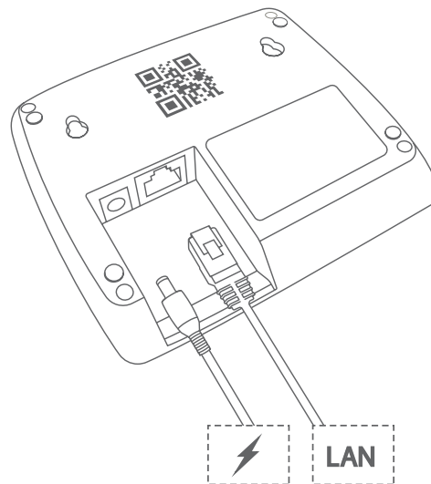
Abbildung 5: Homematic IP Access Point anschließen
